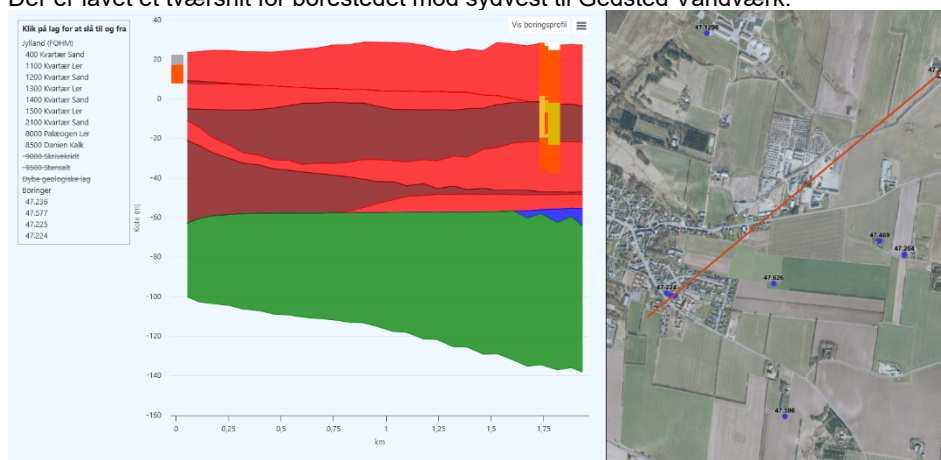
Figur 4 - Tværsnit mod sydvest
