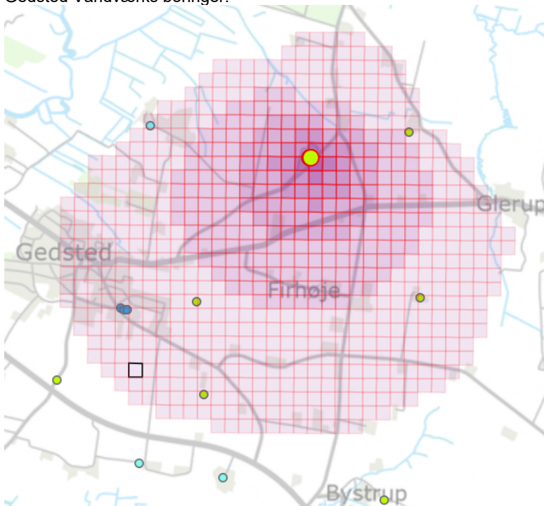
Figur 6 – Sænkningstragt for indvinding af grundvand for markvandning
