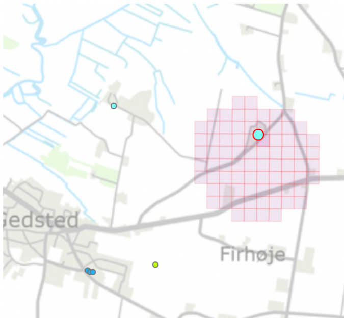
Figur 5 - Sænkningstragt for indvinding af grundvand til driften
