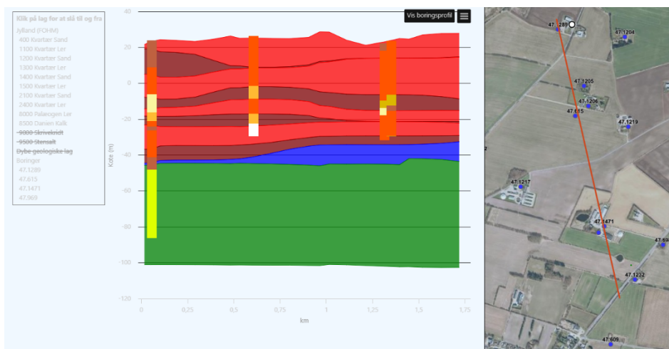
Figur 2 - Tværsnit mod syd
