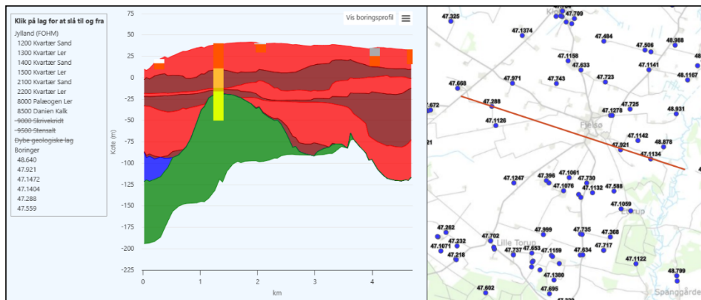
Figur 1 - Tværsnit fra Simested Å gennem boringen mod Korsvejen.
