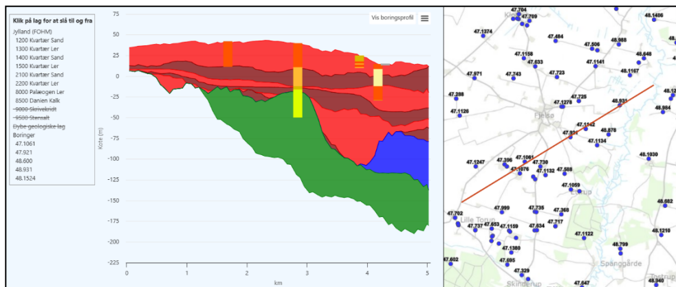
Figur 2 - Tværsnit fra Lille Torupvej gennem boringen mod Simested Å.
