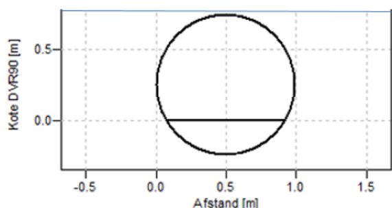
Figur 5.1 Rørbrø hvor \frac{1}{4} af røret er under regulativmæssig bund. Eksempel Ø100 cm rør, hvor 0,25 m ligger under regulativmæssig bund.
