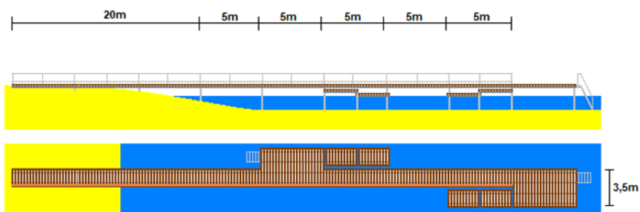
Planskitse
