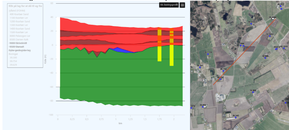
Figur 2 - Tværsnit mod nordøst
