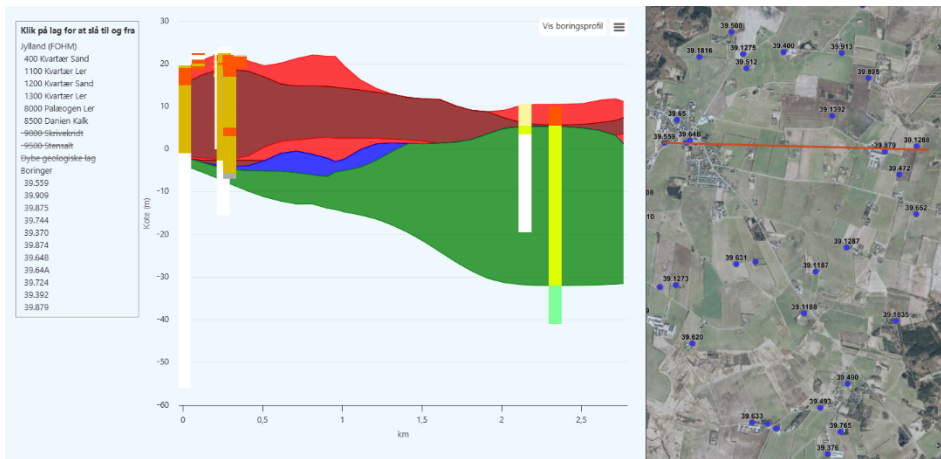
Figur 3 - Tværsnit mod øst
