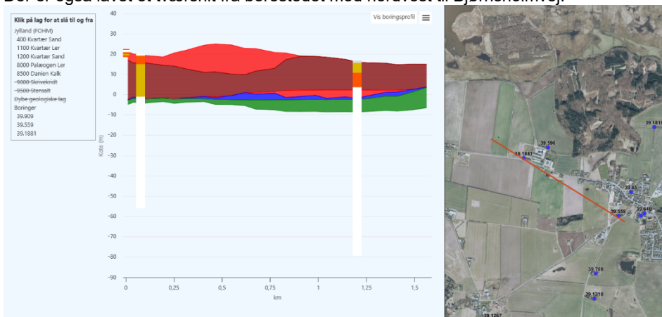
Figur 4 - Tværsnit mod nordvest
