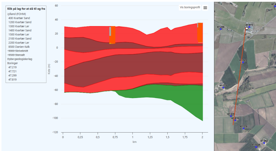
Figur 3 - Tværnsnit mod syd
