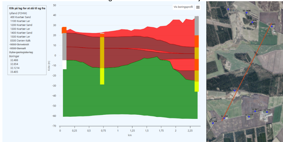
Figur 1 - Tværsnit mod nordøst
